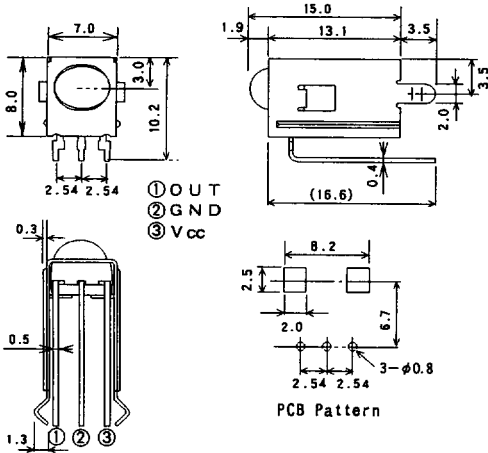
NJL64H000 UNIT : mm
