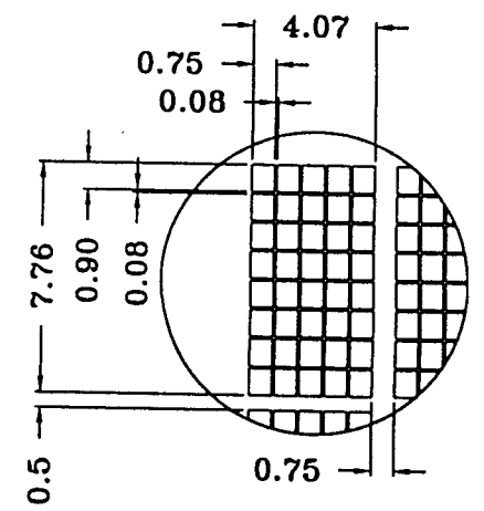
DETIAL A:
