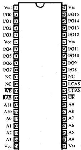
42 SOJ
