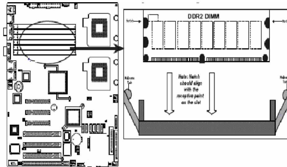
图2.4-2 内存模块位置示意图
