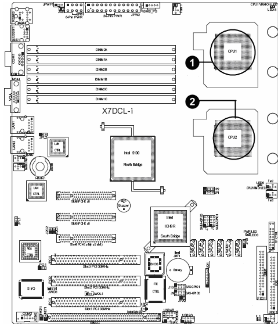
图2.4-1 CPU 单元位置示意图
