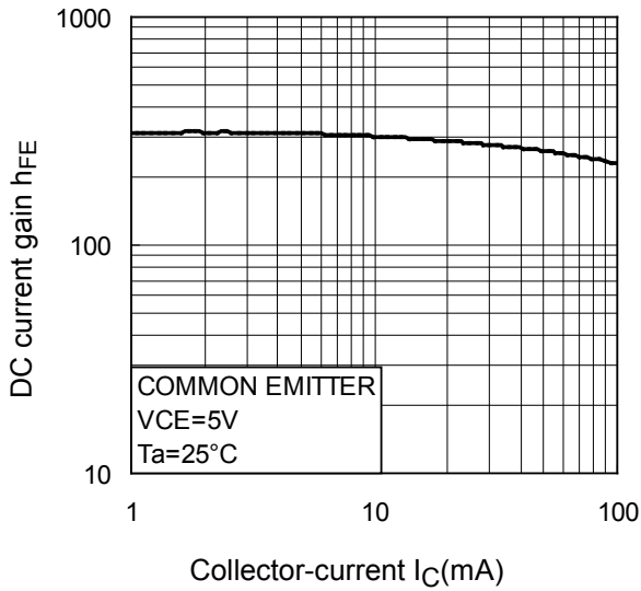
h_{FE}-I_C
