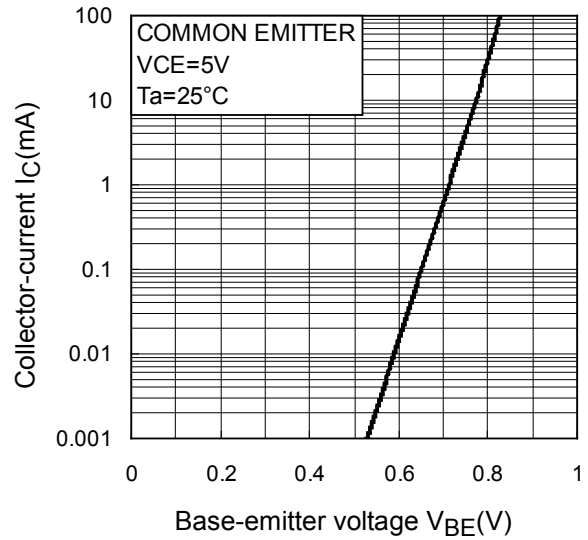
I_C-V_{BE}
