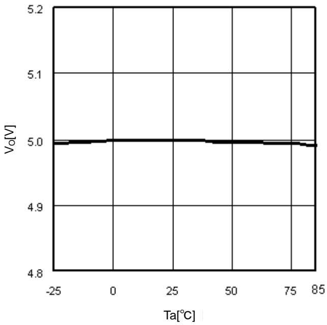
Fig.9 T_a-V_O ( I_o=0mA )
