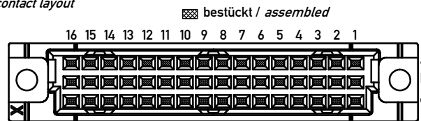
Bestückungsplan / contact layout
