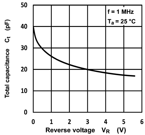
Fig. 8.2 C_t - V_R
