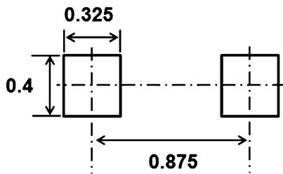
fSC(SOD-923) (unit: mm)
