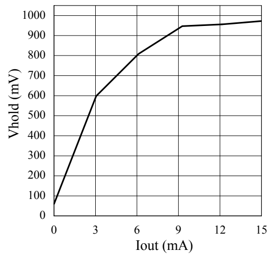
Vhold-Iout
