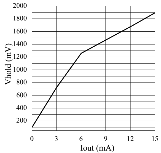
Vhold-Iout
