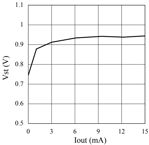
Vst-Iout
