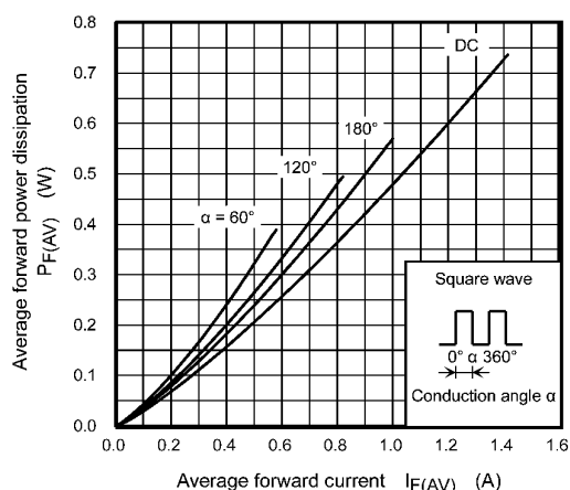
Fig. 10.2 P_{F(AV)} - I_{F(AV)}
