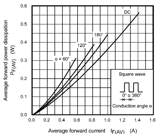
Fig. 10.2 P_{F(AV)} - I_{F(AV)}
