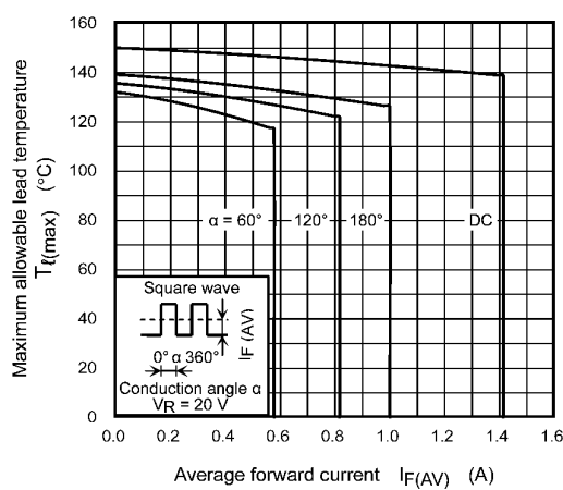
Fig. 10.4 T_{l(max)} - I_{F(AV)}
