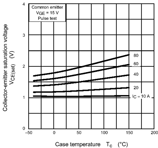
Fig. 8.5 V_{CE(sat)} - T_C
