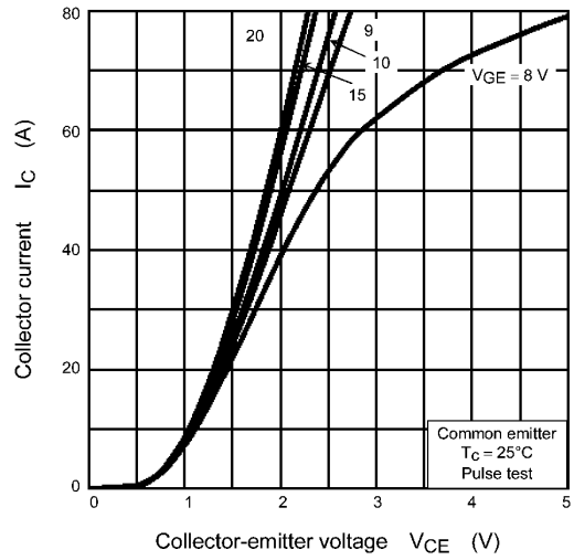
Fig. 8.2 I_C - V_{CE}
