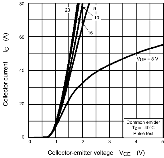
Fig. 8.1 I_C - V_{CE}
