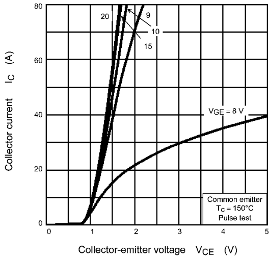
Fig. 8.3 I_C - V_{CE}
