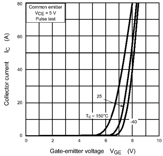
Fig. 8.4 I_C - V_{GE}
