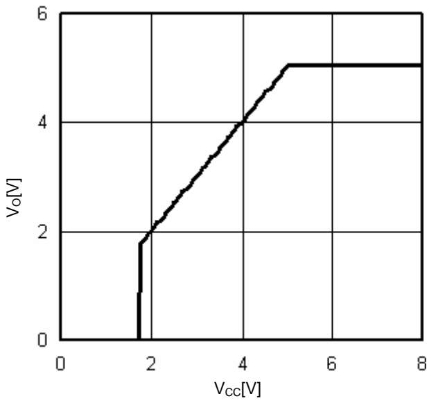
Fig.15 V CC -V O (I O =0mA)
