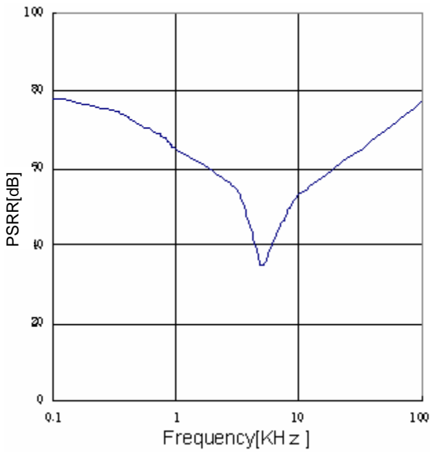
Fig.21 PSRR( I_o=0mA )
