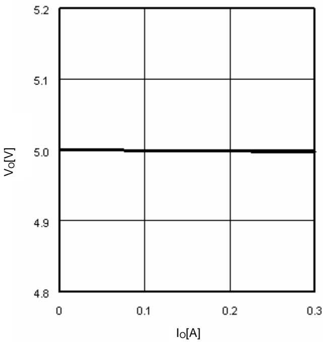
Fig.13 I_o - V_o
