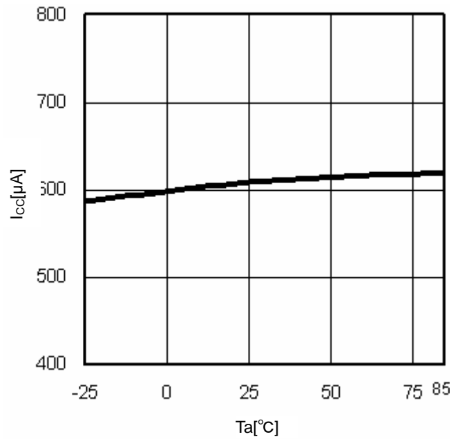
Fig.10 T a -I CC
