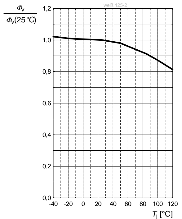
Relative Lichtstrom 1) 2) Seite 23 Relative Luminous Flux 1) 2) page 23 \Phi_V/\Phi_V(25\text{ °C}) = f(T_j) ; I_F = 700\text{ mA} ; ultra white
