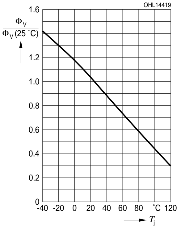
Relative Lichtstrom 1) 2) Seite 23 Relative Luminous Flux 1) 2) page 23 \Phi_V/\Phi_V(25\text{ °C}) = f(T_j) ; I_F = 700\text{ mA} ; true green
