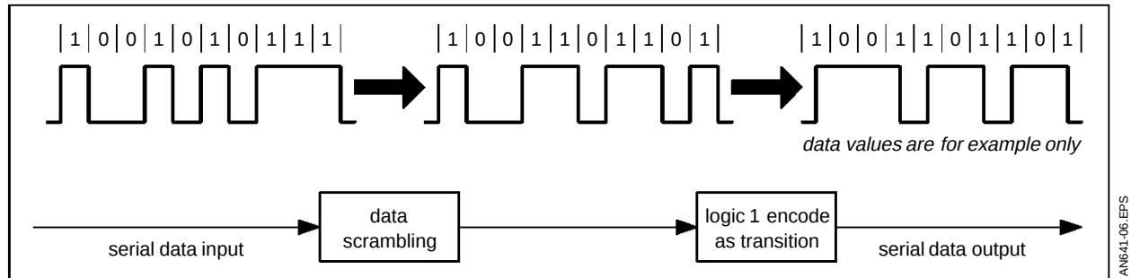
Figure 6 : Data Serialisation
