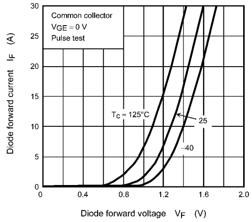
Fig. 8.14 I_F - V_F
