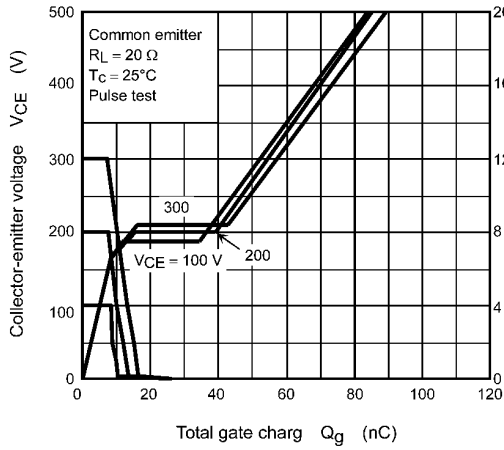
Fig. 8.13 V_{CE} , V_{GE} - Q_g
