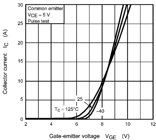
Fig. 8.5 I_C - V_{GE}
