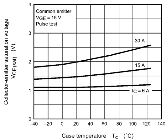
Fig. 8.6 V_{CE}(\text{sat}) - T_C
